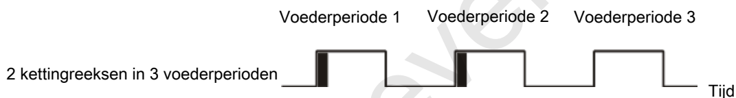
Figuur 9: Kettingvoeding: Voorbeeld 2: Verdeling van het aantal kettingreeksen
